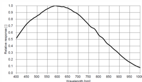
MV-CA020-10UM 量子效率
