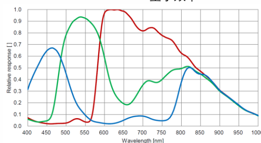
MV-CA020-10UC 量子效率
